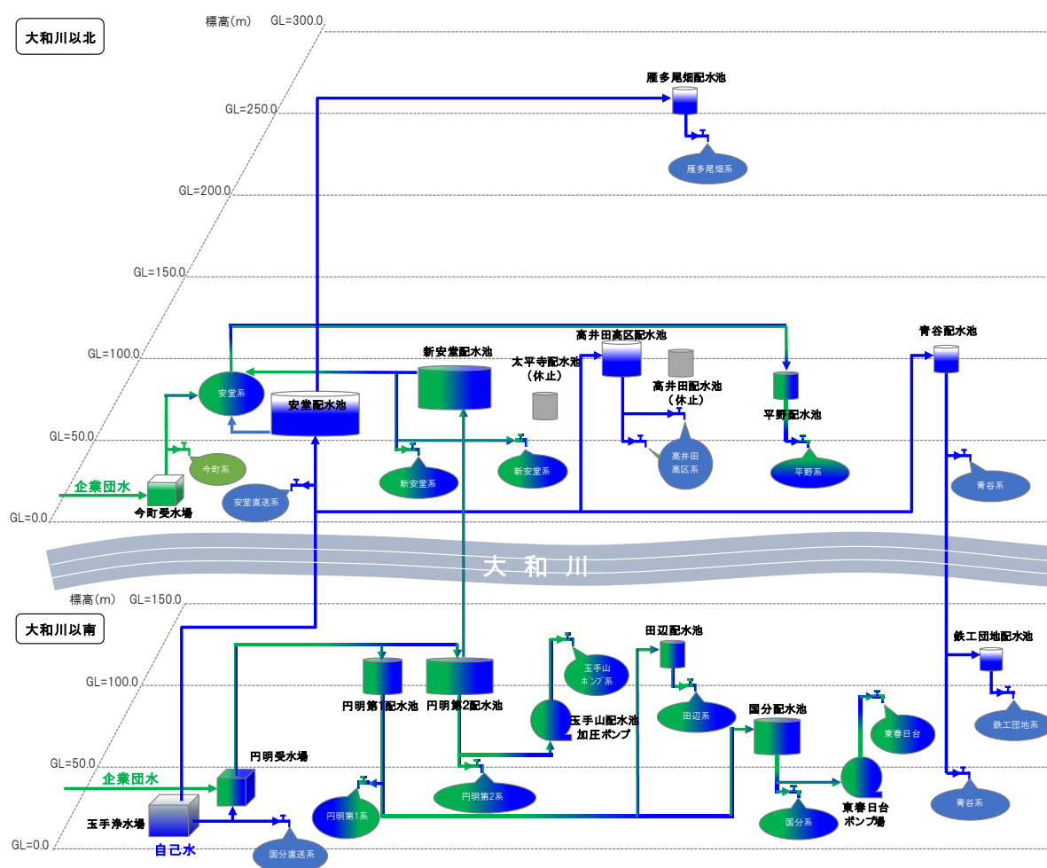
図3 送配水系統図
