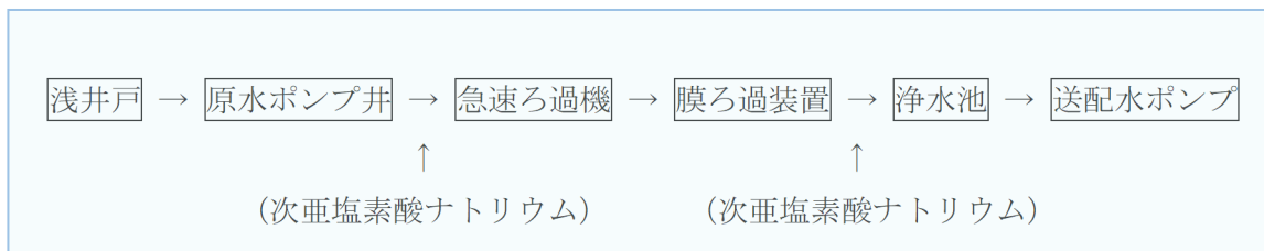
図 1 玉手浄水場の浄水処理フロー
